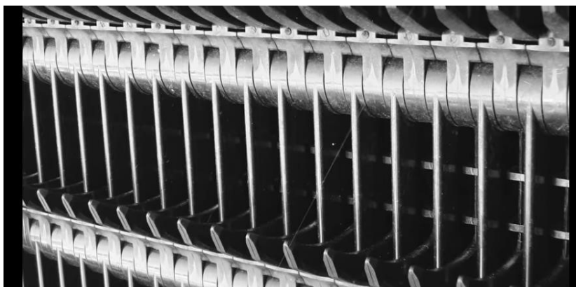
Detalhe do encaixe preciso do elemento filtrante entre os eixos horizontais grade esteira existente.
